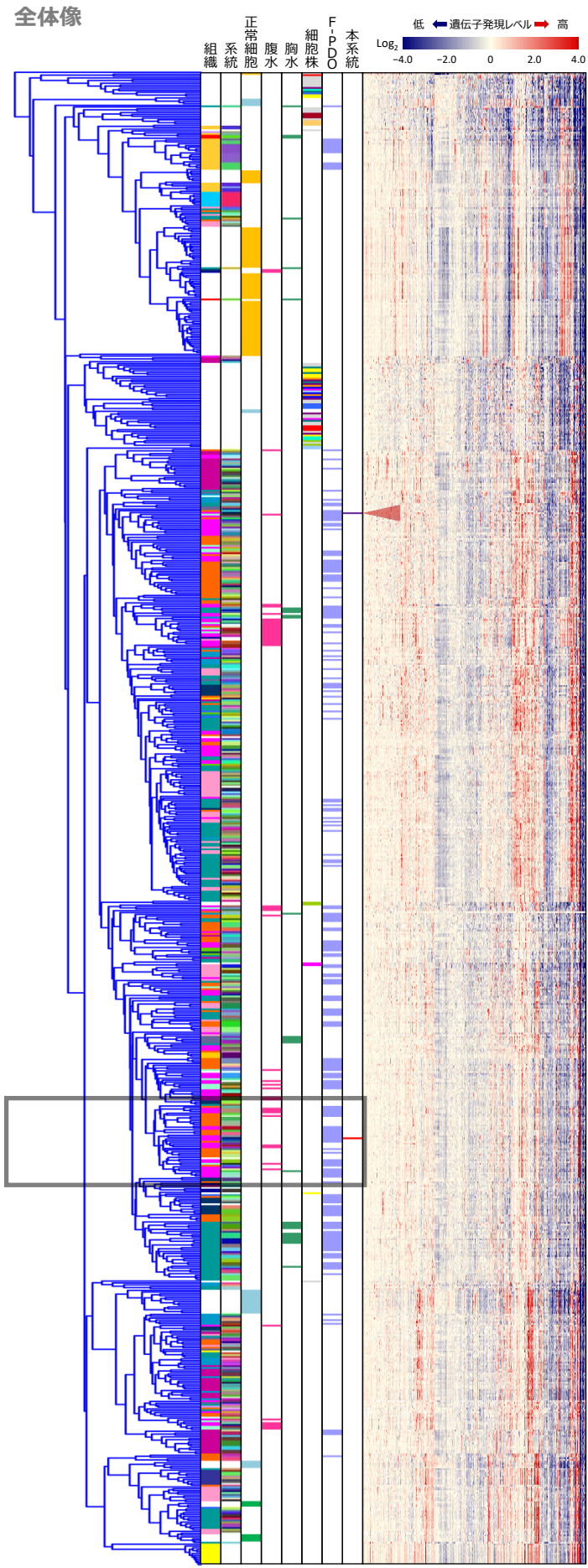
発現変動が大きい遺伝子群 (2,135 transcripts)
